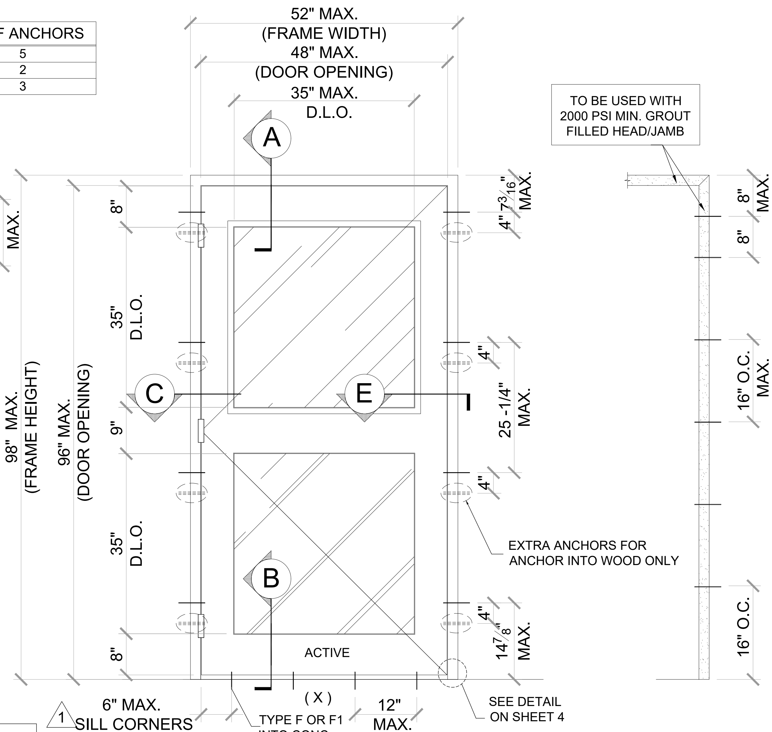
SINGLE DOOR TYP. EXT. ELEVATION
