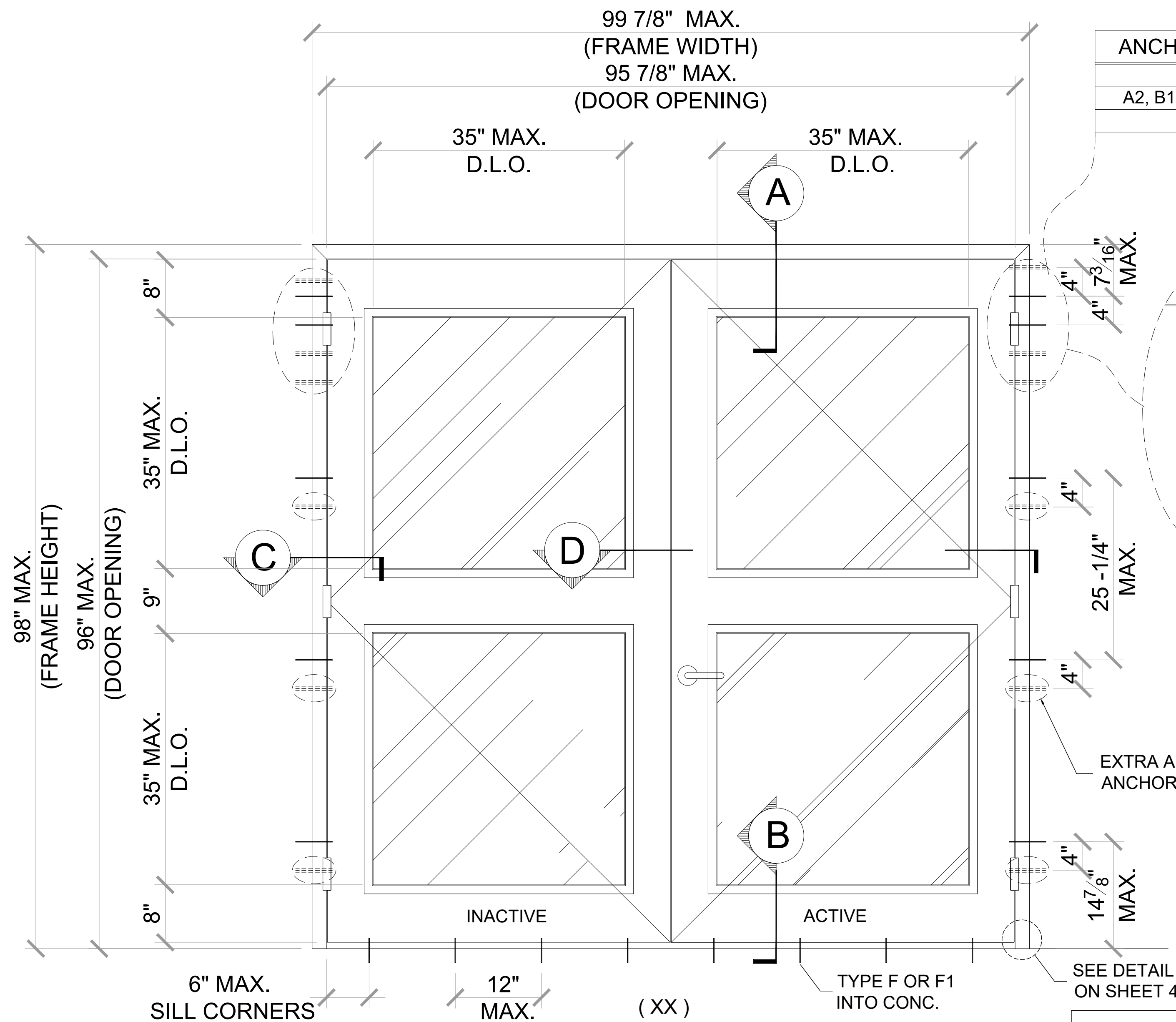
DOUBLE DOOR TYP. EXT. ELEVATION
